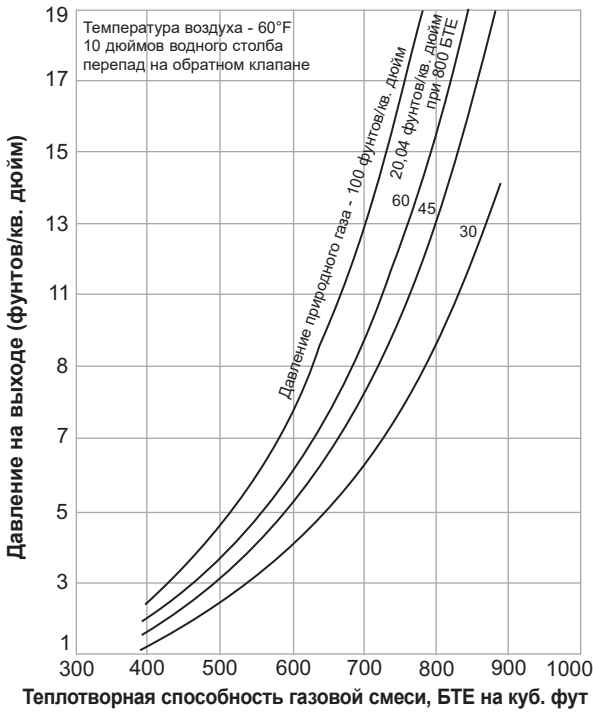
График U - Кривые противодействия смеси природного газа и воздуха
