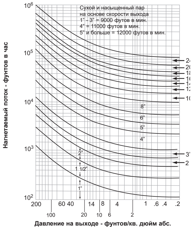
График С - Соотношения мощности паровых струйных термокомпрессоров с рабочим горячим паром 125 фунтов/кв. дюйм.
