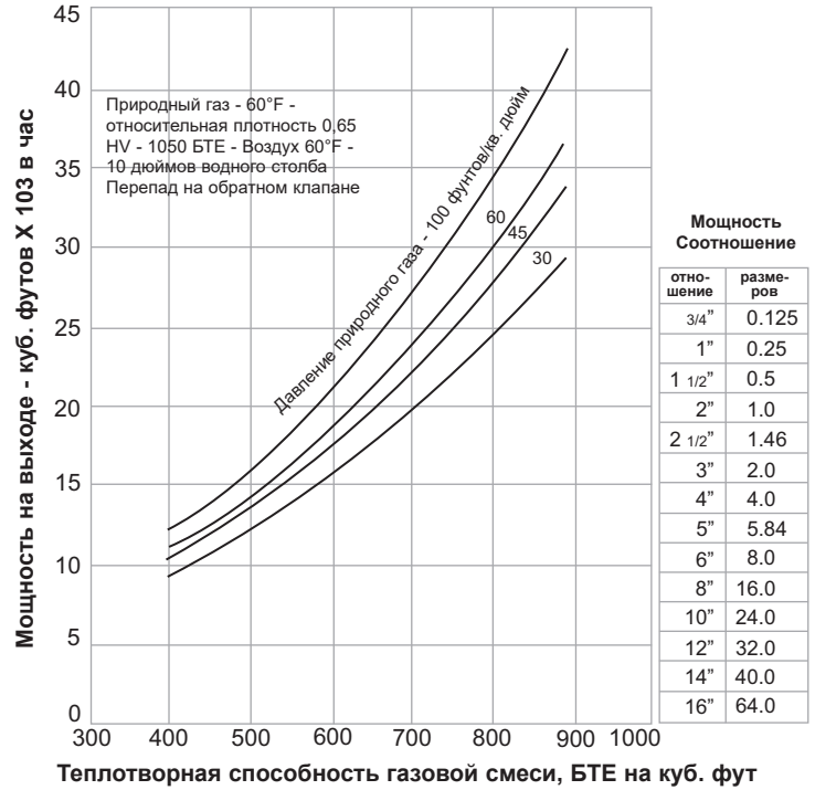
График X - Кривые мощности воздушной смеси для 2-дюймовых воздушных струйных компрессоров типа 420
